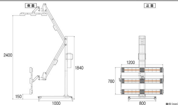
図面 製造元:有限会社 テクノ製作所
