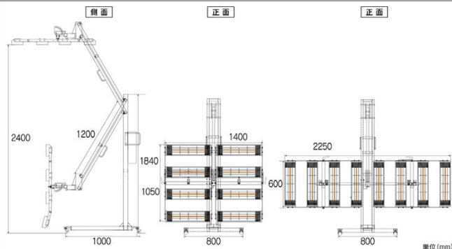
図面 製造元:有限会社 テクノ製作所
